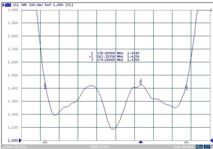
Courbe TOS
