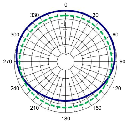
Espacement quart d'onde horizontal
