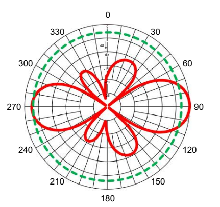
Espacement demi-onde vertical
