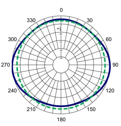
Espacement demi-onde horizontal
