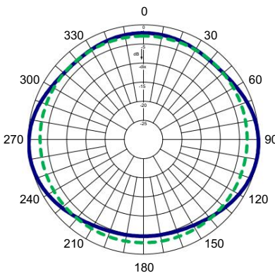
Espacement demi-onde horizontal
